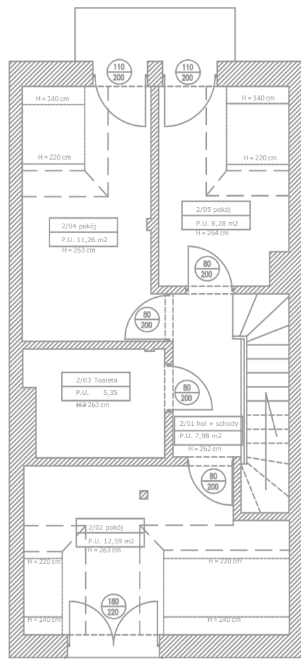
RZUT PIĘTRA
